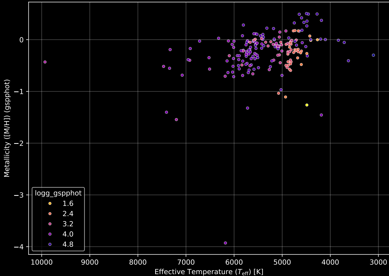
APOGEE DR17 Field: [195+32_MGA] Stellar Population Parameters (n= 197)
